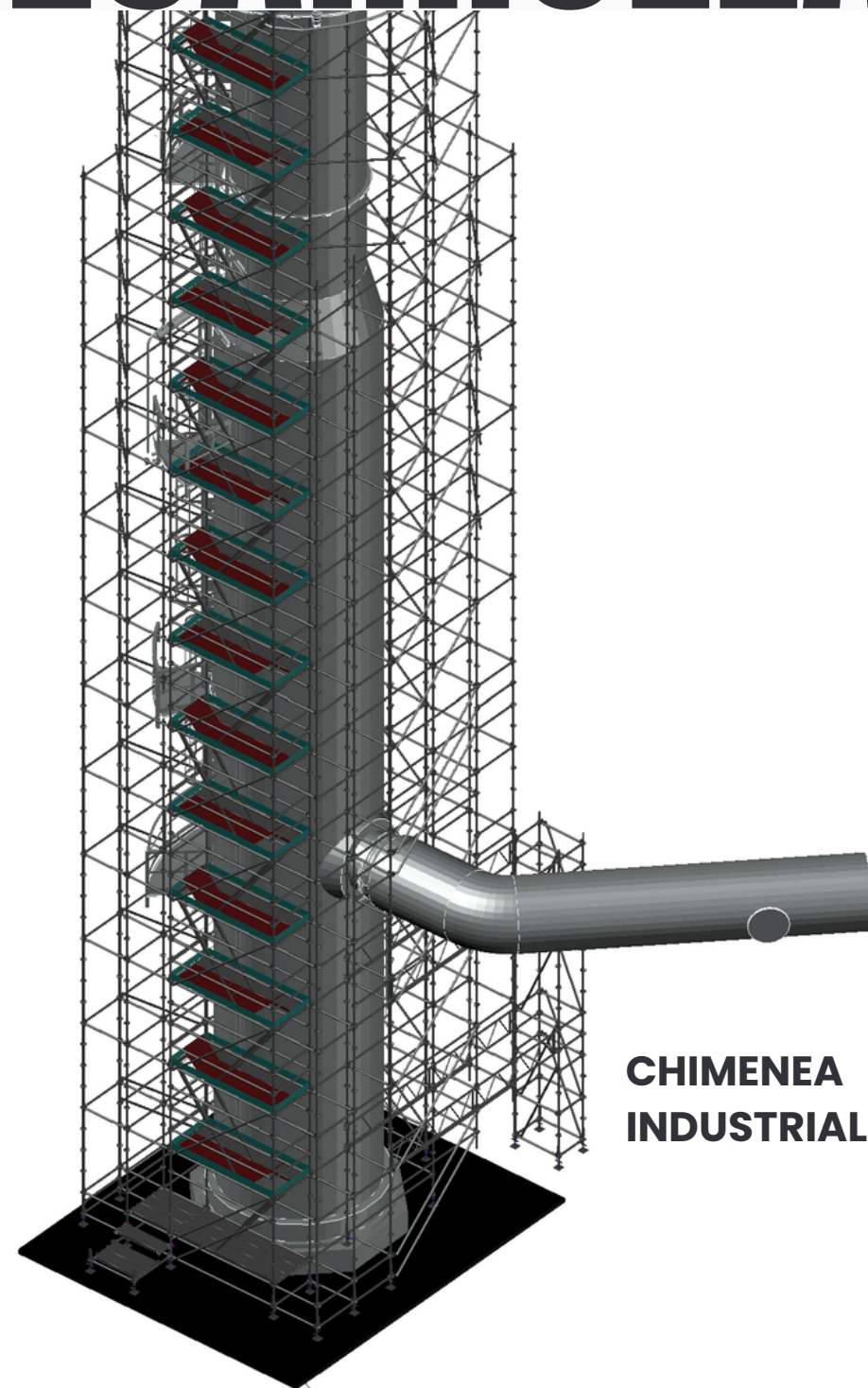
TORRE ANCLADA
